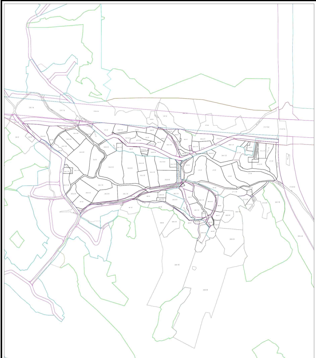
수산4지구 지적재조사 완료지구 지형도면 (변경 전)
