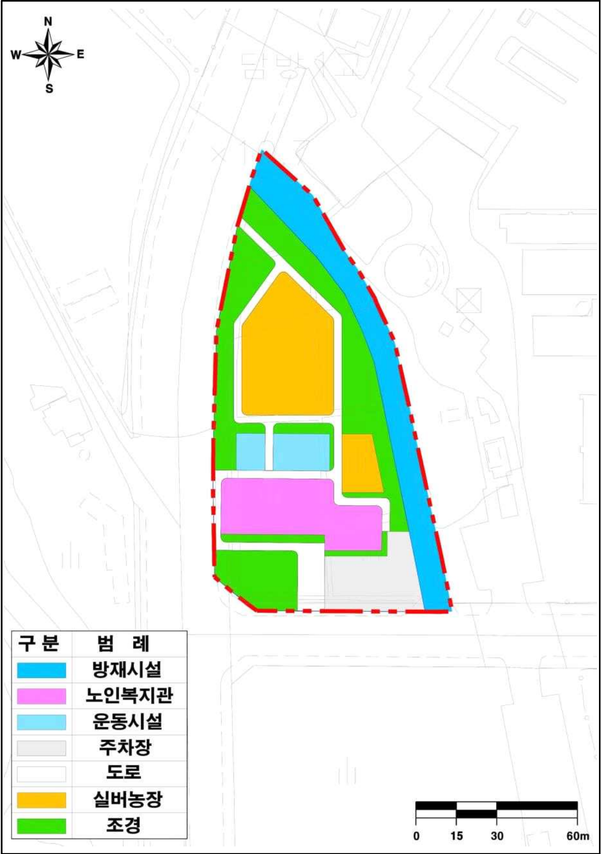
(그림 1-2) 토지이용계획도
